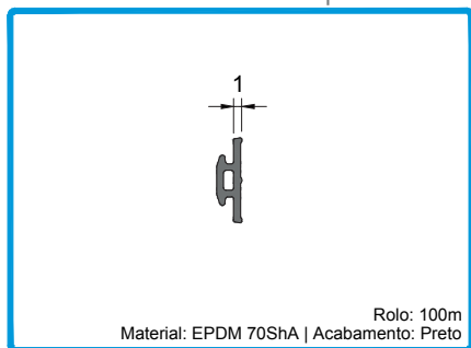
208014 JUNTA VD 2122 PRT Rolo: 100m Material: EPDM 70Sha | Acabamento: Preto
