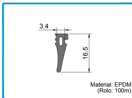
208249 JUNTA VD 2099 Material: EPDM (Rolo: 100m)
