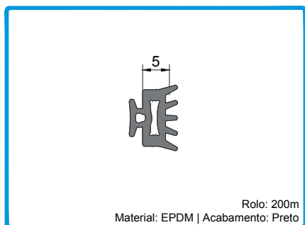
208427 JUNTA VD 2068 Rolo: 200m Material: EPDM | Acabamento: Preto
